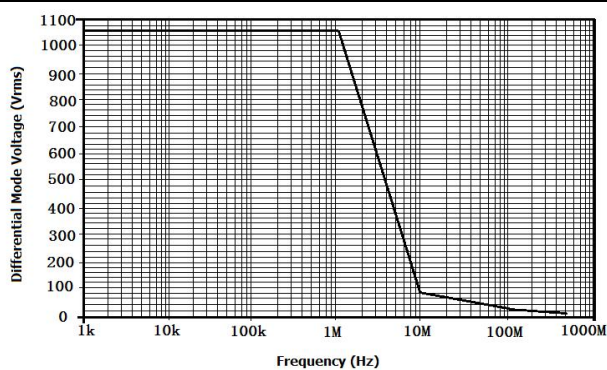
8 图 2 DP6150B 最大差模电压 VS 频率
